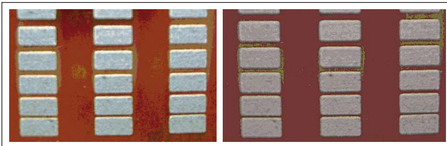
Bild 2: Konturenstabilität bei RT und nach 150 °C/5 min (kleinster Abstand 0,1mm)
